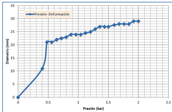
Figura 9. Relación presión-deformación diametral.
