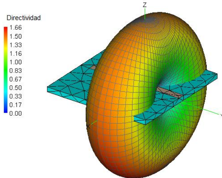
Figura 4. Desempeño de la antena monopolo
