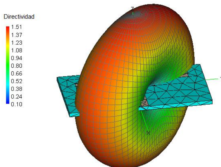
Figura 8. Desempeño de la antena dipolo plano resonante
