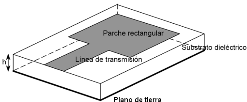
Figura 1. Antena parche rectangular
